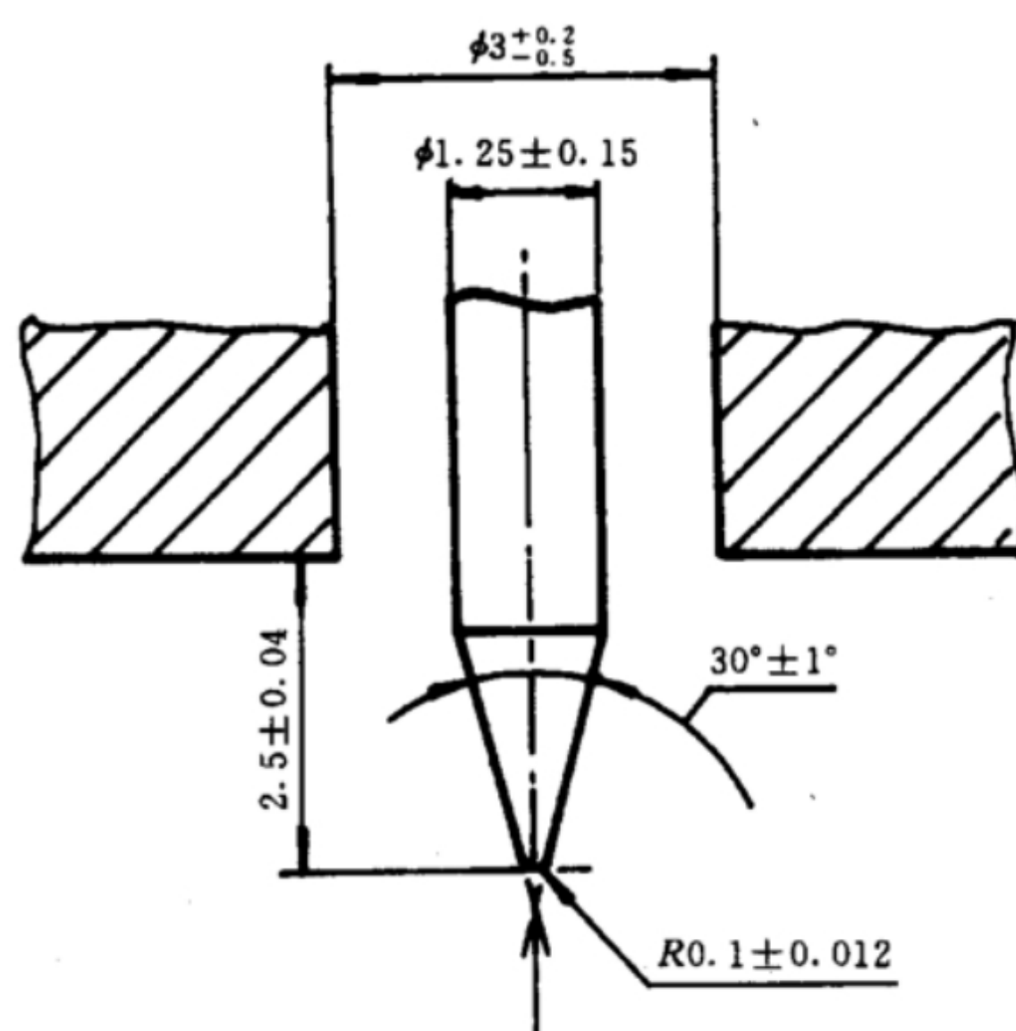
图 2 邵氏 D 型硬度计压针
