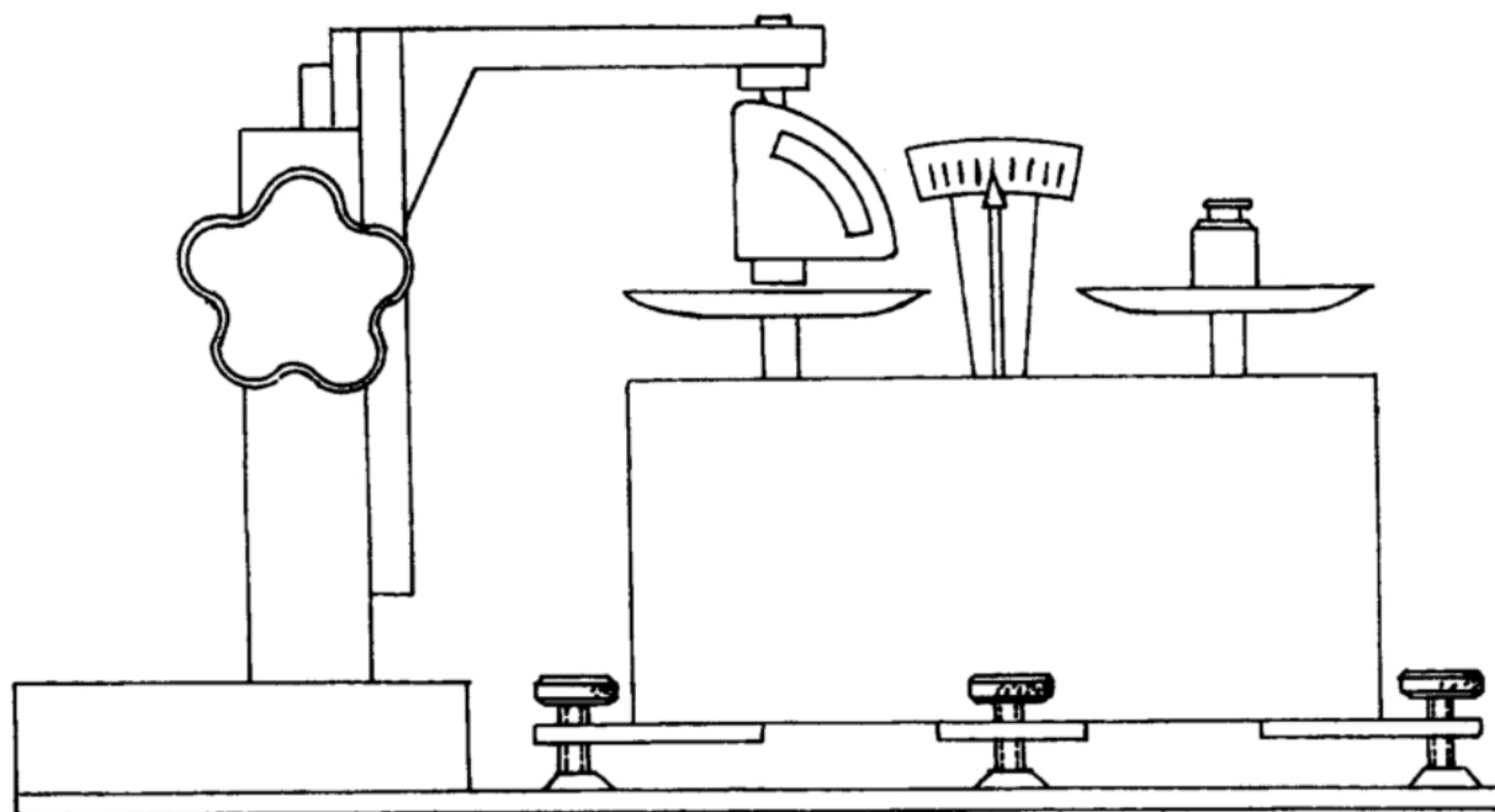
图 3 邵氏硬度计试验力校准装置
