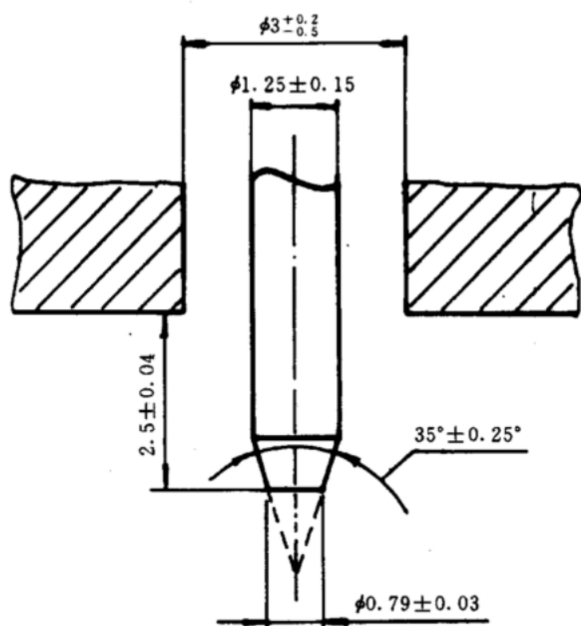
图 1 邵氏 A 型硬度计压针
