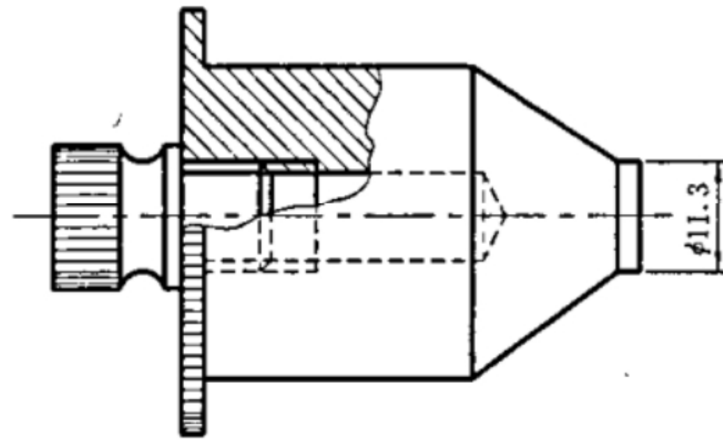
图 7 干燥试验器示意图
