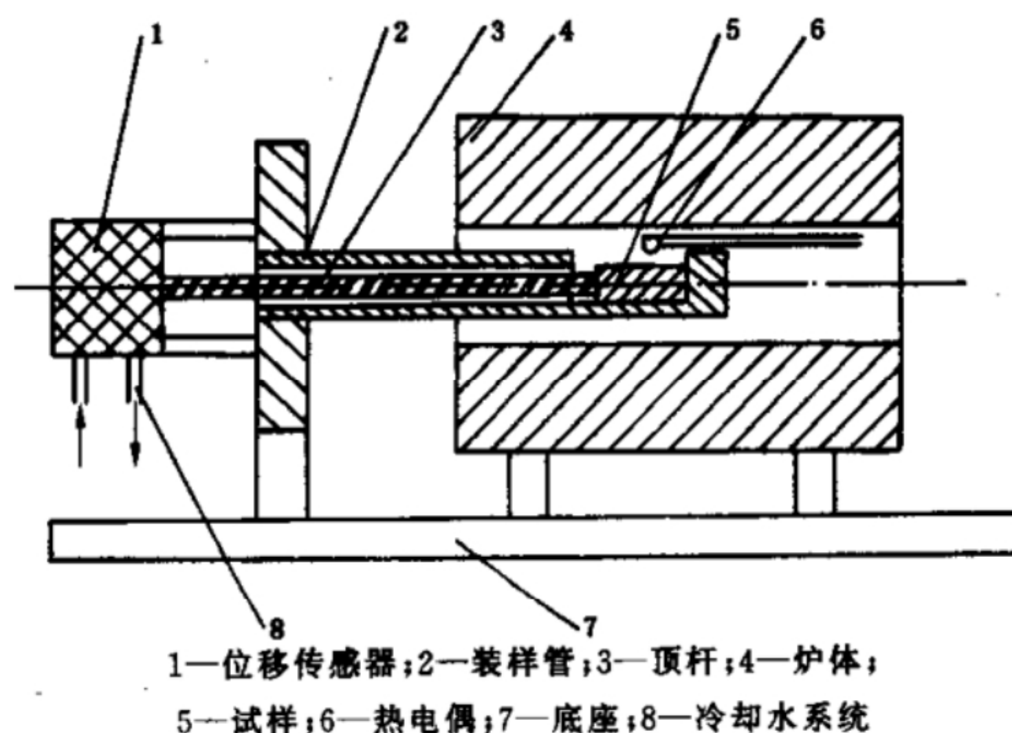
图 1 测量装置示意图
