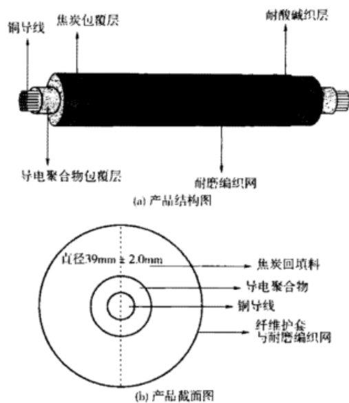
图 2 导电聚合物线性阳极示意图
