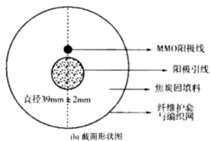
图 1 MMO/Ti 线性阳极示意图
