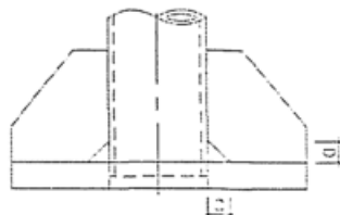
图 4.2.5-1 加劲肋切角
