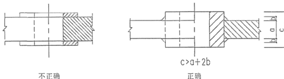
图 4.2.5-3 热镀锌的零构件的加强拉耳板、螺栓孔加强板构造
