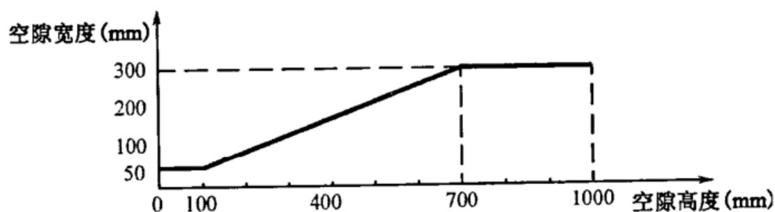
图 1 型钢间的空隙宽度的要求
