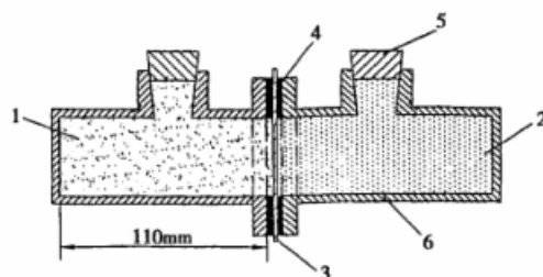
图 C.2.2 涂层抗氯离子渗透性试验装置示意图
