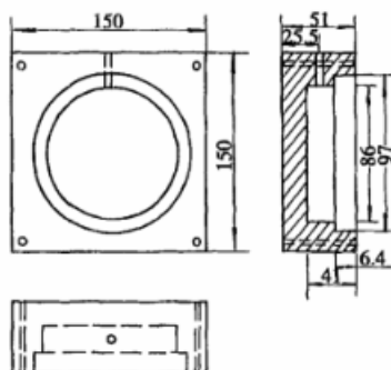
图 B.3.2 试验槽结构图(mm)
