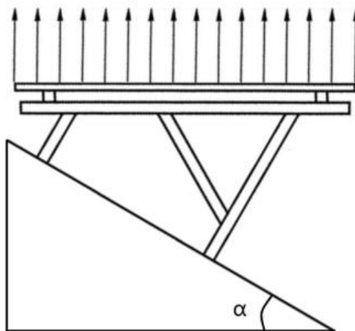
图 A.2 垂直组件面静载荷变形试验示意图
