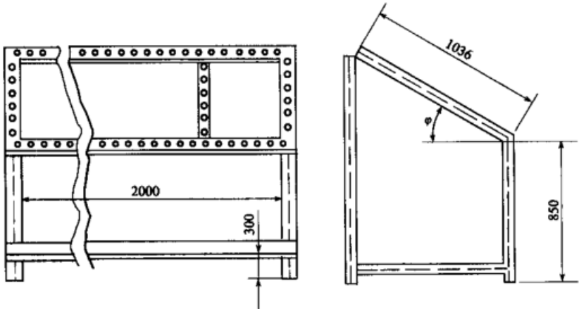
骨架全部采用 30mm×4mm 的角钢 φ—曝露角度
