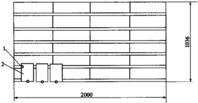
图 1-1 曝露架面 1—瓷绝缘子;2—试验样板
