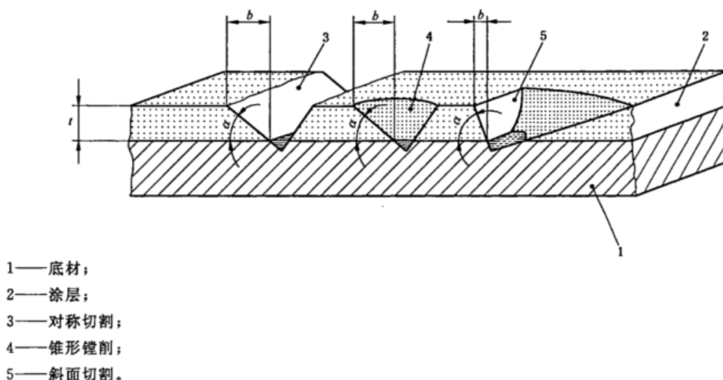
图 12 对称切割、锥形镗削和斜面切割
