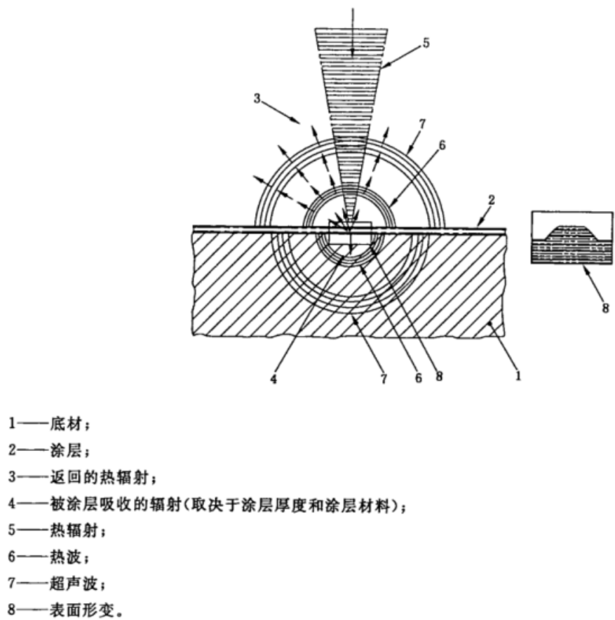
图 4 光热厚度测量法中辐射与试样的相互作用(显示表面形变)
