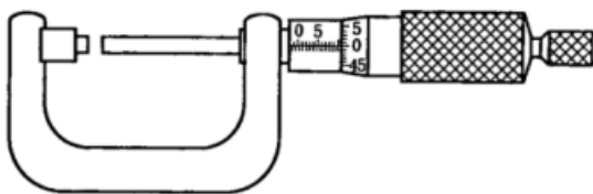
图 5 外卡规测微计
