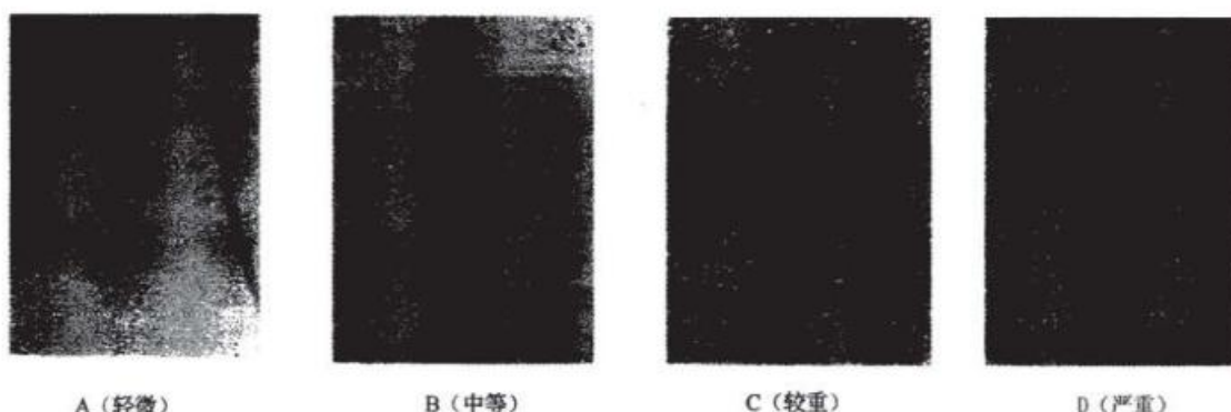
图 3 盐雾试验后样板表面漆膜起泡图例
