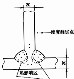
图 A.7 断面宏观检查试样
