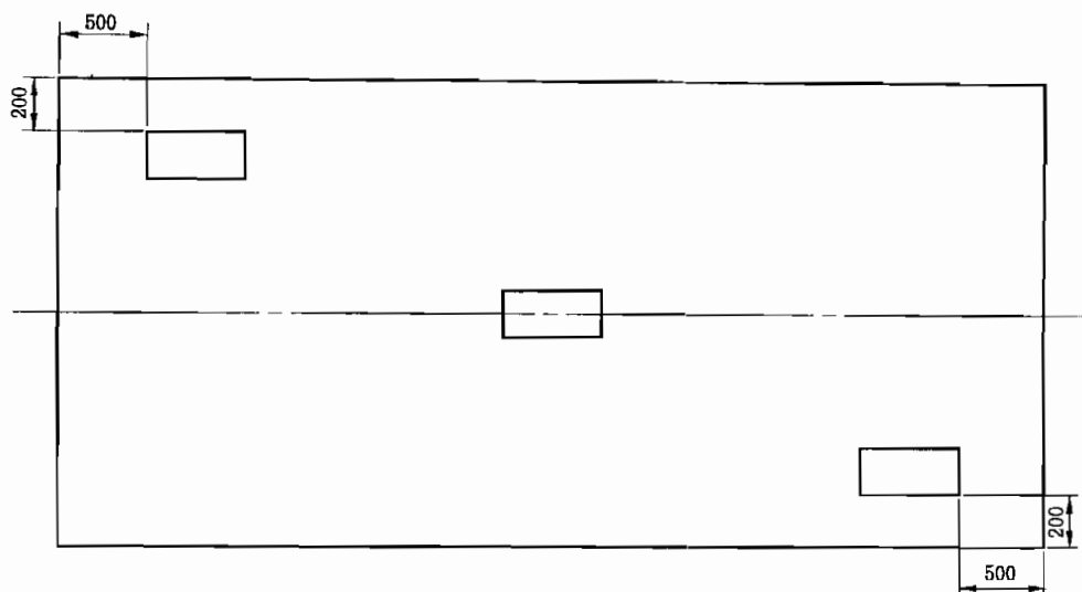
图 A.1 检验板粘贴位置
