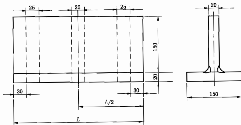
图 A.6 角焊接试样截取图
