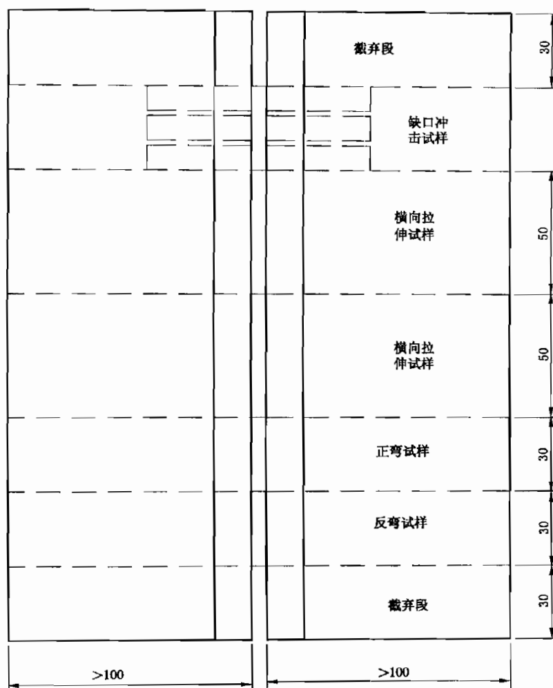
图 A.2 对焊接试样截取图
